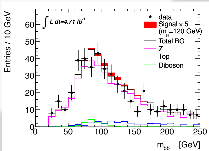
ZH->llbb: No p_T > 45\text{GeV} cut
