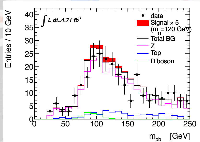
ZH->llbb: with p_T > 45\text{GeV} cut
